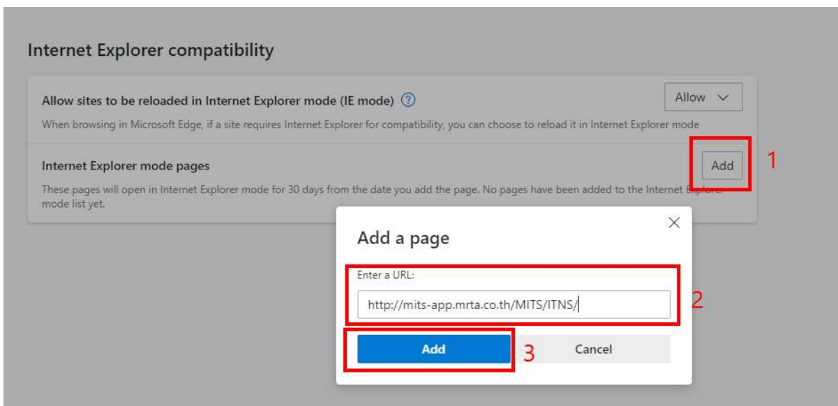
รูปที่ 6 การเพิ่มหน้า page ให้รองรับ IE mode
